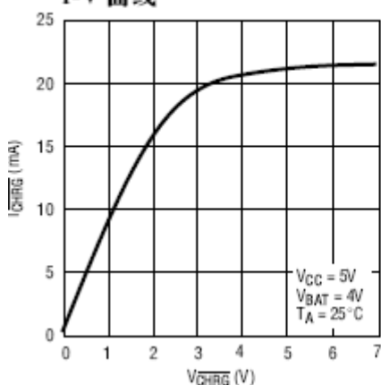
强下拉状态下的 \overline{CHRG} 引脚 I-V 曲线
