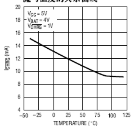
强下拉状态下 \overline{CHRG} 引脚电流与温度的关系曲线
