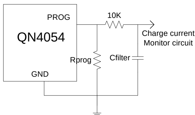
图3 隔离PROG脚上的容性负载和滤波电路
