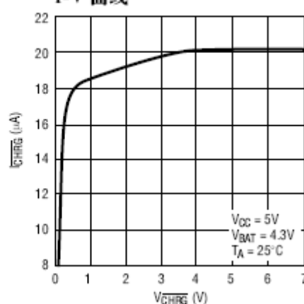
弱下拉状态的 \overline{CHRG} 引脚 I-V 曲线
